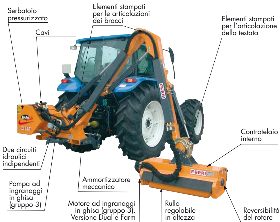
Sistema floating
