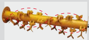
Rotore elicoidale "OVERLAP" a doppia elica con coltelli sovrapposti
