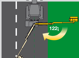
Sistema di massima sicurezza con ritorno automatico tramite accumulatore di azoto (SRA)
